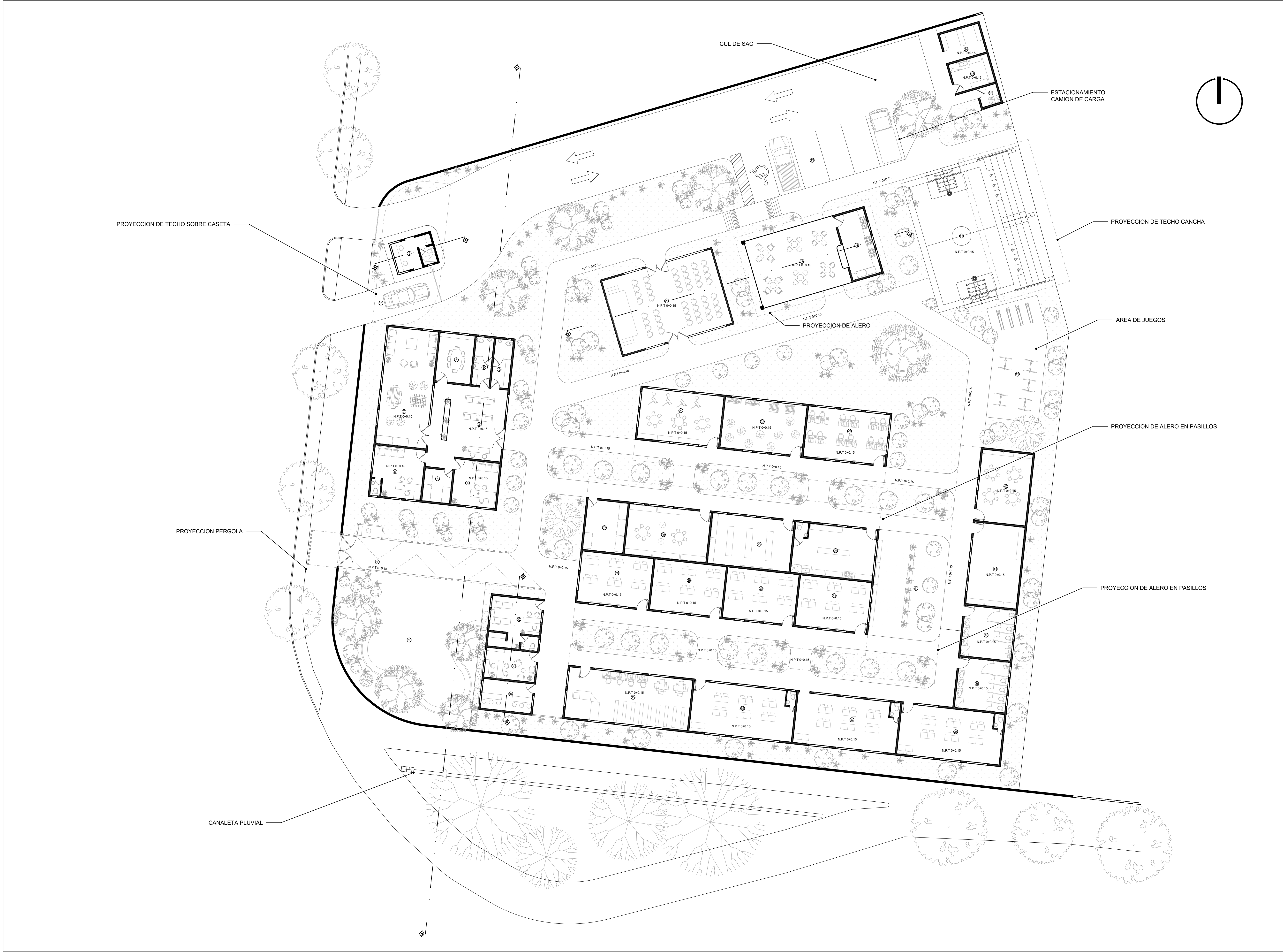
PLANTA ARQUITECTONICA CENTRO ESCOLAR EUGENIA DUEÑAS ESC 1:175
