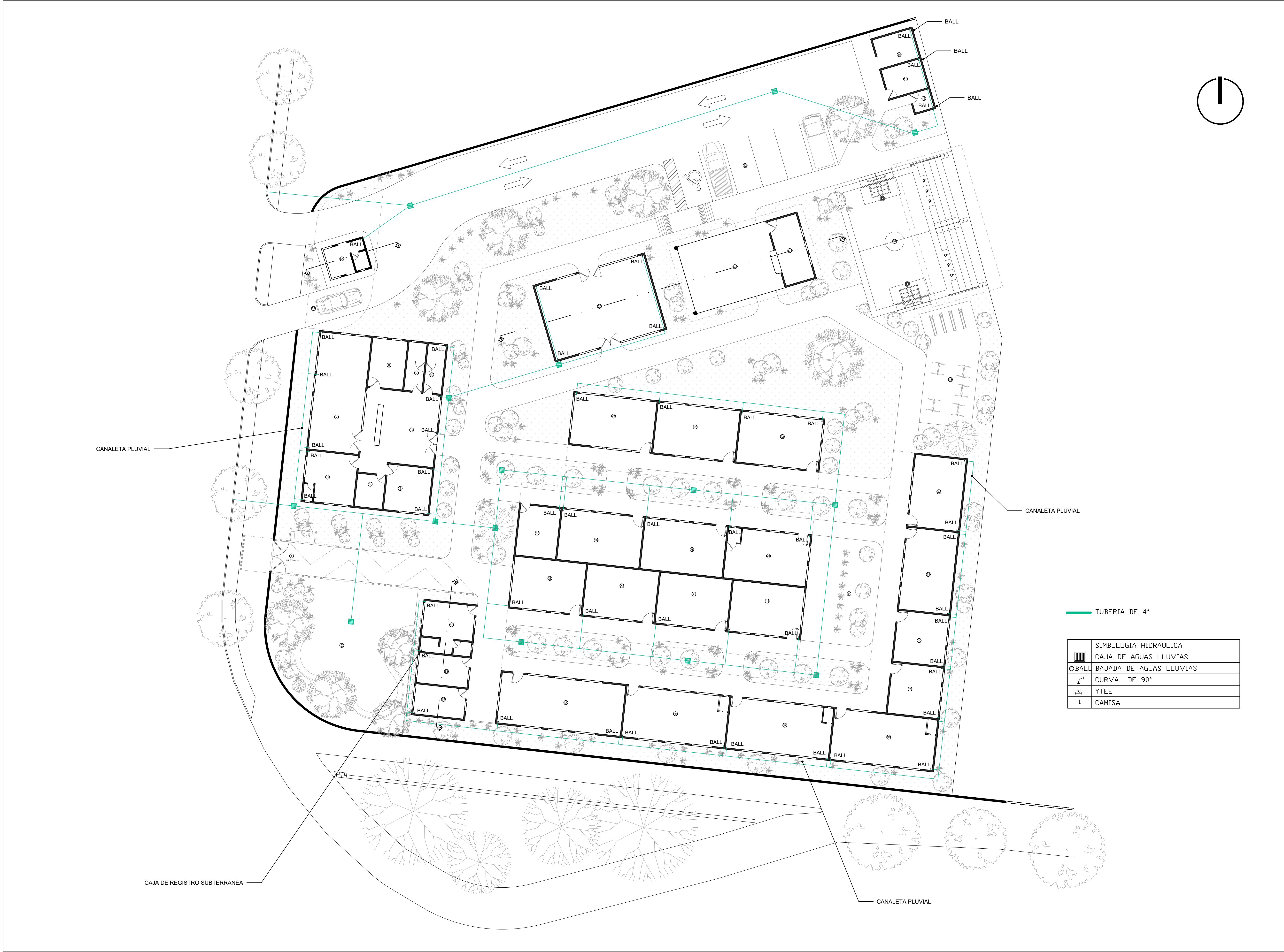
PLANTA DE AGUAS LLUVIAS ESC 1:175
